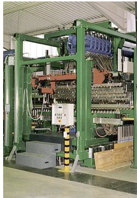
Abschreckstation
